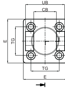
ÇB: Çatal Bağlantı Piston rod clevis mounting
