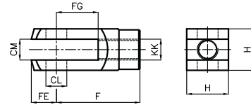
ÇB: Çatal Bağlantı Piston rod clevis mounting
