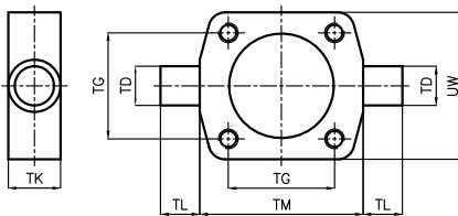
OEB: Orta eklem bağlantı Trunnion mounting
