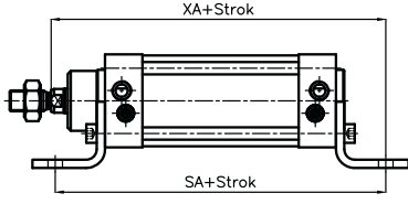
Ayak bağlantı Foot mounting
