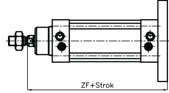
Arka flanş bağlantı Rear flange mounting
