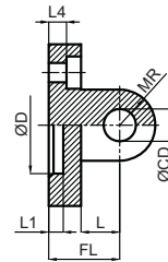
EB: Eklem bağlantı Swivel flange mounting
