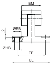
EYB: Yer bağlantı Clevis foot
