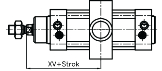
Orta eklem bağlantı Trunnion mounting
