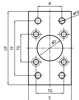
EB: Eklem bağlantı Swivel flange mounting
