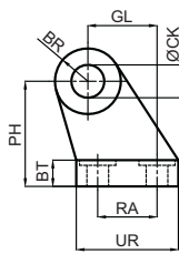
EYB: Yer bağlantı Clevis foot
