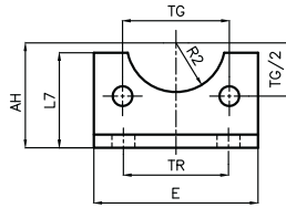
AB: Ayak bağlantı Foot mounting
