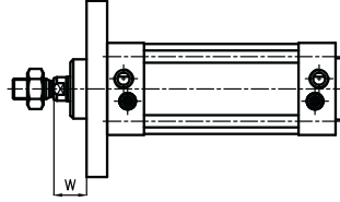
Ön flanş bağlantı Front flange mounting
