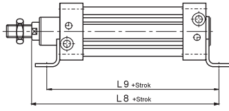
Ayak bağlantı Foot mounting
