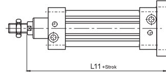
Arka flanş bağlantı Rear flange mounting
