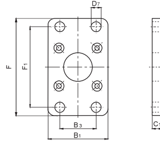
FB: Flanş bağlantı Flange mounting
