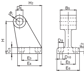
YB: Yer bağlantı Clevis foot
