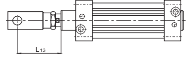
Çatal bağlantı Piston rod clevis mounting
