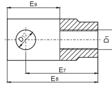
ÇB: Çatal bağlantı Piston rod clevis mounting
