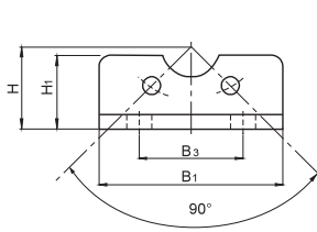
AB: Ayak bağlantı Foot mounting
