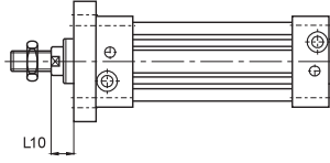
Ön flanş bağlantı Front flange mounting
