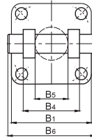
EB: Eklem bağlantı Swivel flange mounting
