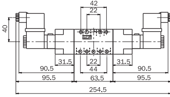
Yatık Bobinli Valf Horizontal type solenoid SV-1/4-5/2-B-B-Y
