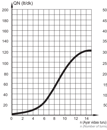
FKV 1/8
