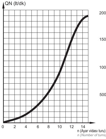
FKV 1/4
