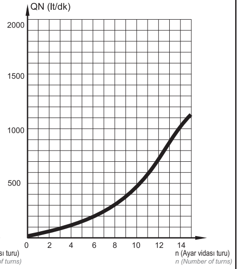
FKV 1/2
