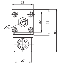
BOBİN KAPAĞININ ÜSTTEN GÖRÜNÜŞÜ
