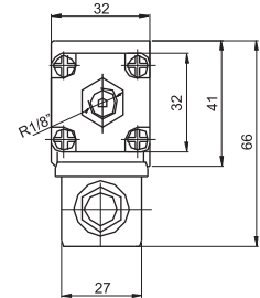
BOBİN KAPAĞININ ÜSTTEN GÖRÜNÜŞÜ
